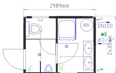
10-и футовый сантехнический блок-контейнер
