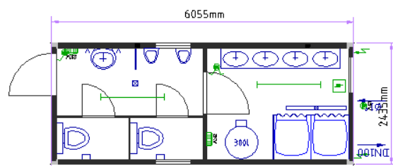
20-и футовый сантехнический блок-контейнер
