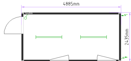
16-и футовый офисный блок-контейнер
